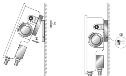
Рис. 5-6 Установка зарядной станции на стену
