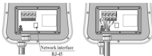
Рис. 5-5 Подключение входного силового кабеля
