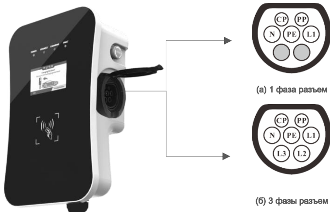
Рис. 3-3 Схема разъема Type 2 на зарядных станциях серии M3B
